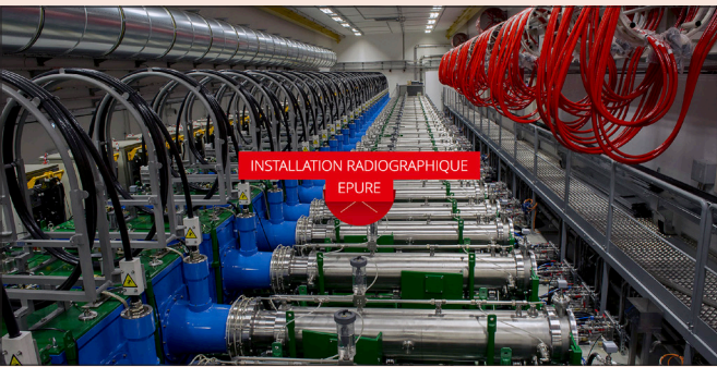
L'un des axes de radiographie éclair du site Epure. Crédit : dam.cea.fr
